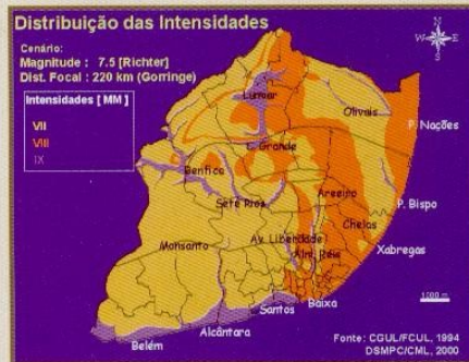
FIG.3 - CARTA DE INTENSIDADES DE LISBOA
