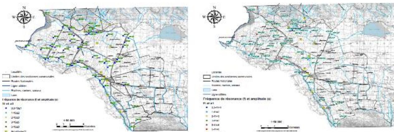
FIG. 22: Carte de fréquences de resonances. A gauche les fréquences f_0 et a_0 et à droite les f_1 et a_1 .
